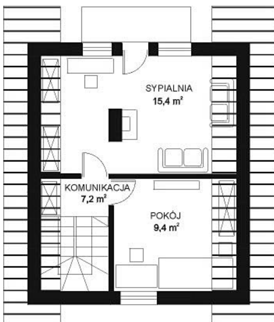
rzut poddasza
