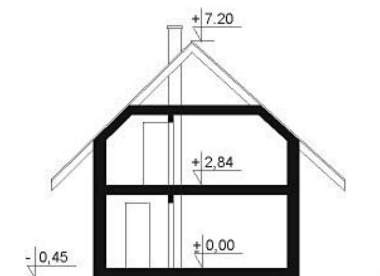
przekrój
