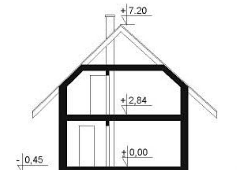
przekrój
